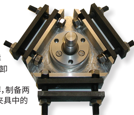
带夹子的试样夹具座
