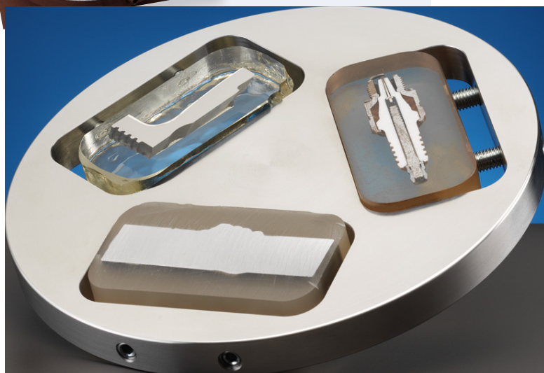
带矩形孔的试样夹具座可以固定长达 70x53 mm 的试样
